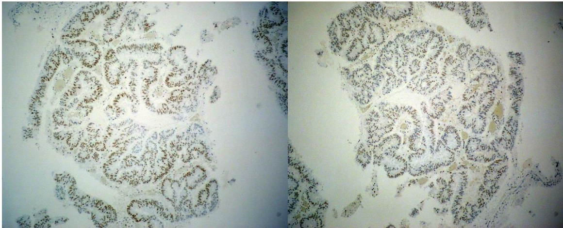
a) MLH1
