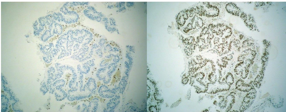
c) MSH6
