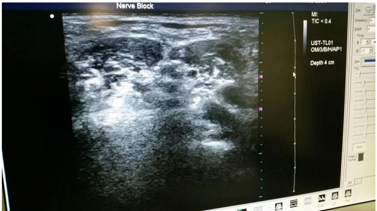
Slika 1.5. Ultrazvučni prikaz interskalenskoga pristupa spletu brahijalnih živaca (fotografirao Marinko Jelečević)
