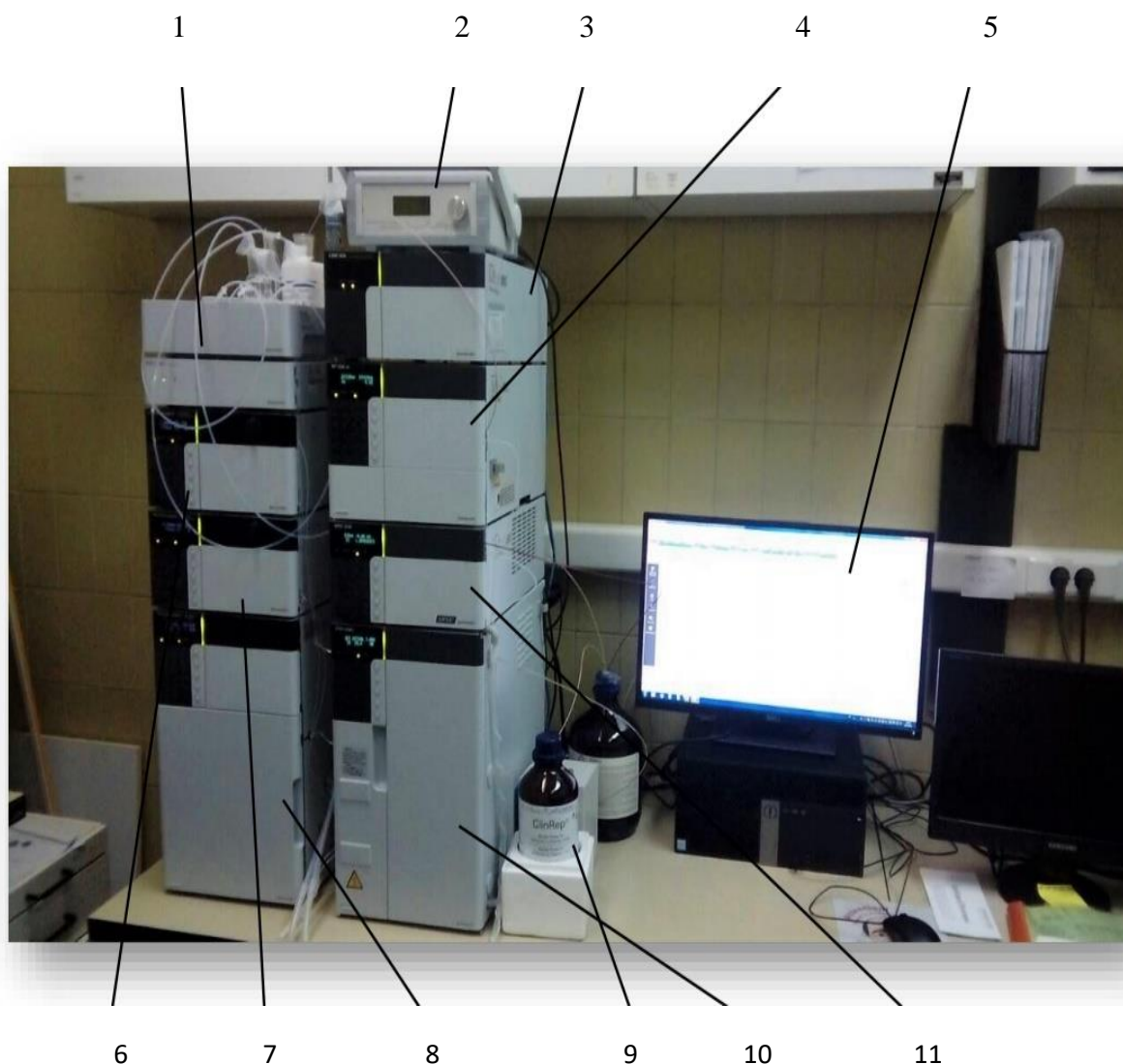
Slika 4. HPLC uređaj. (1- jedinica za otplinjavanje mobilne faze; 2- ECD; 3- komunikacijski modul; 4- FLD; 5- računalo; 6- pumpa A; 7- pumpa B; 8- autoinjektor; 9- mobilna faza; 10- pećnica; 11- UV detektor). Izvor: fotografirala autorica.
